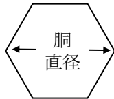
六角吊灯笼寸法
